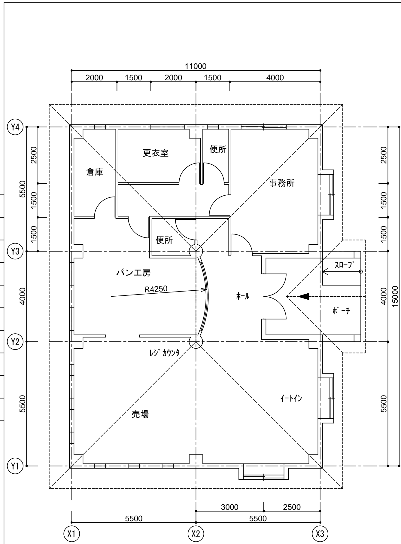
平面図 S=1:100
