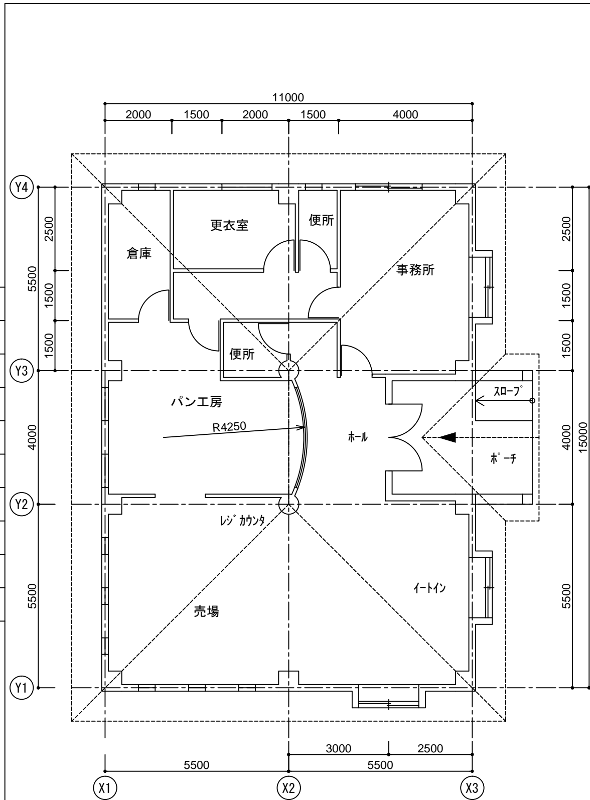
平面図 S=1:100
