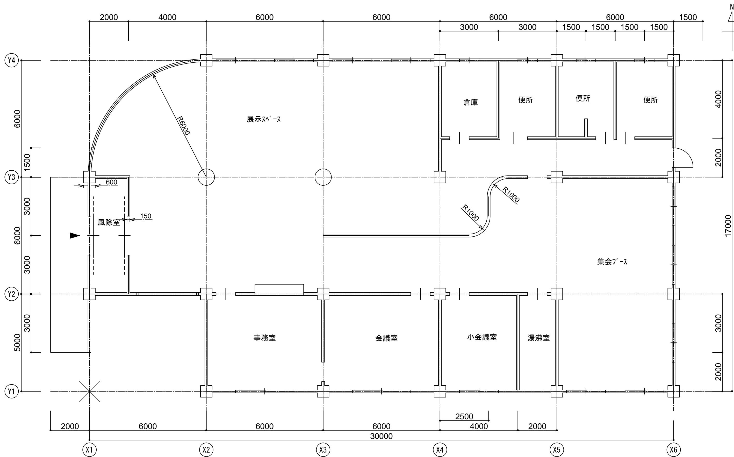
平面図 S=1:100
