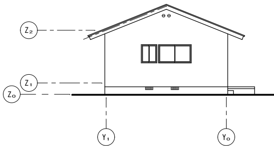
西立面図 (S=1/100)
