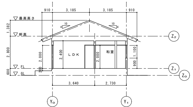
A-A断面図 (S=1/100)
